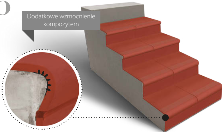
Дополнительное усиление композитом / Додаткове зміцнення композитом.
